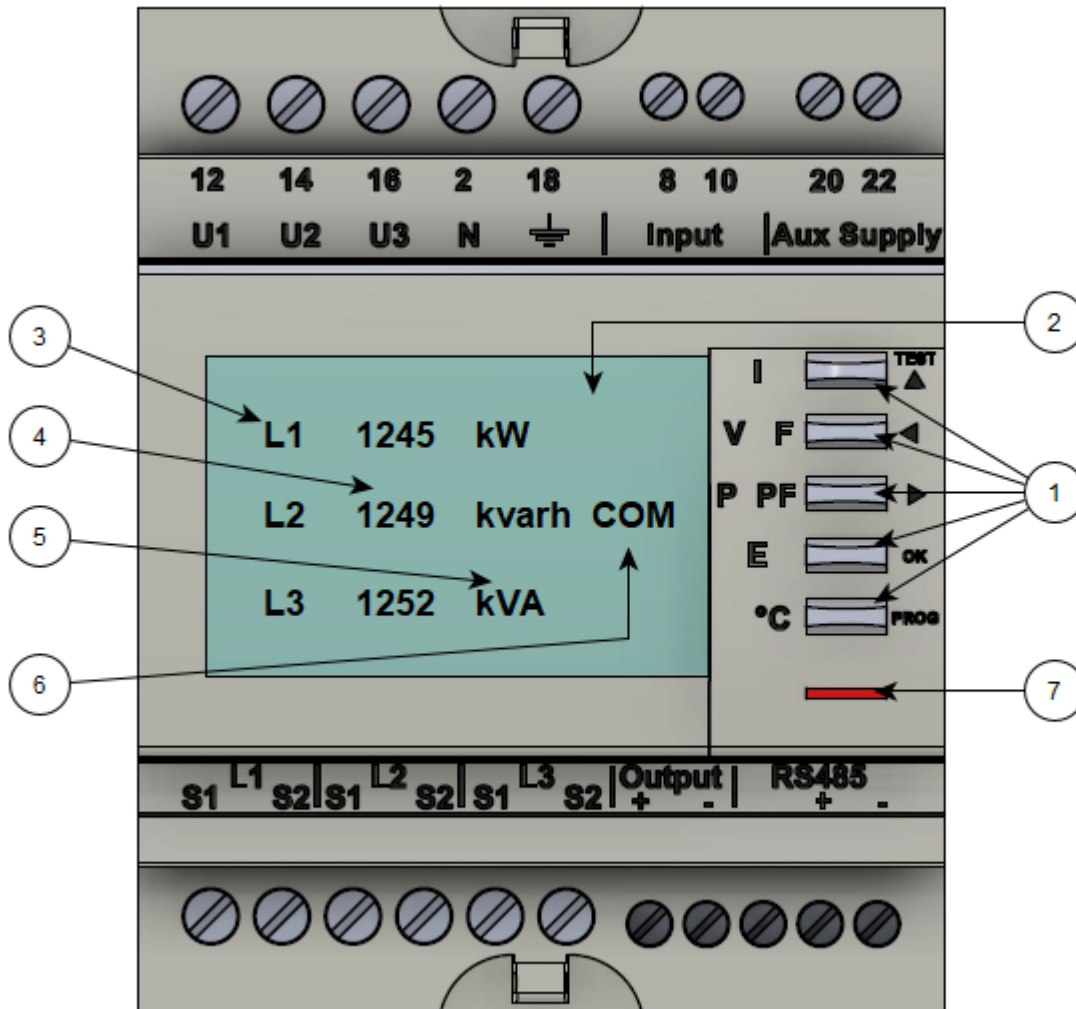
Abbildung 7. Bedienelemente
