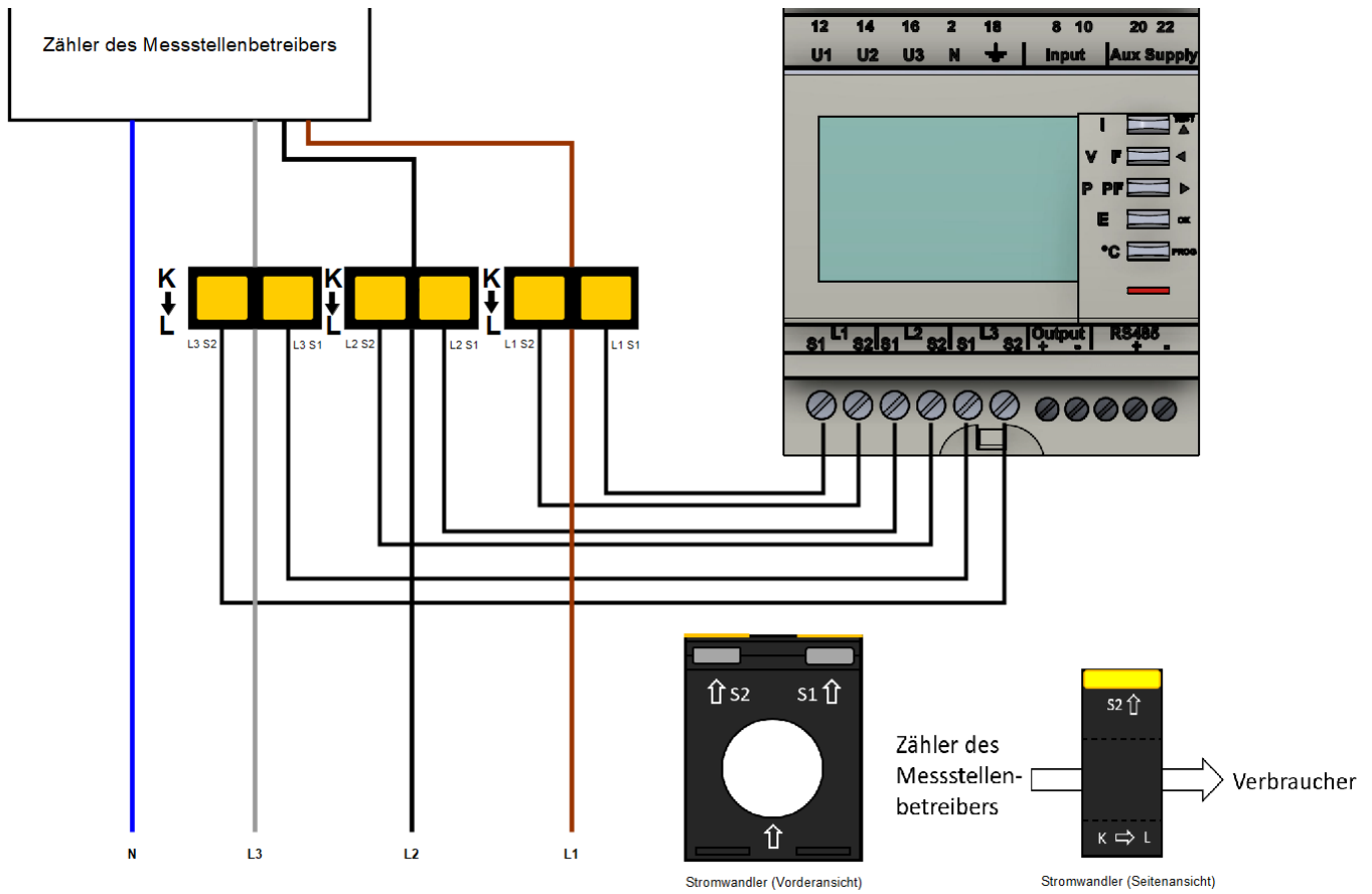
Abbildung 3. Anschluss Stromwandler Zähler Messtellenbetreiber
