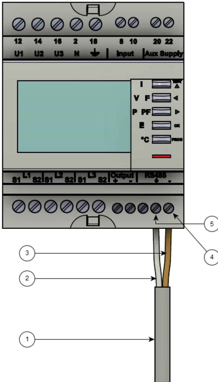
Abbildung 5. Anschluss RS-485
